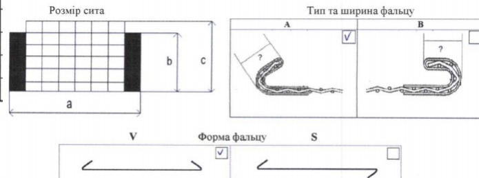
Образец сита с фальцами (вид V) и нахлестом (вариант 2)
